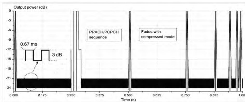
Abbildung 2.4: Schematische Darstellung der Expositionssignalförmigkeiten beim Expositionssystem für UMTS (1950MHz)
