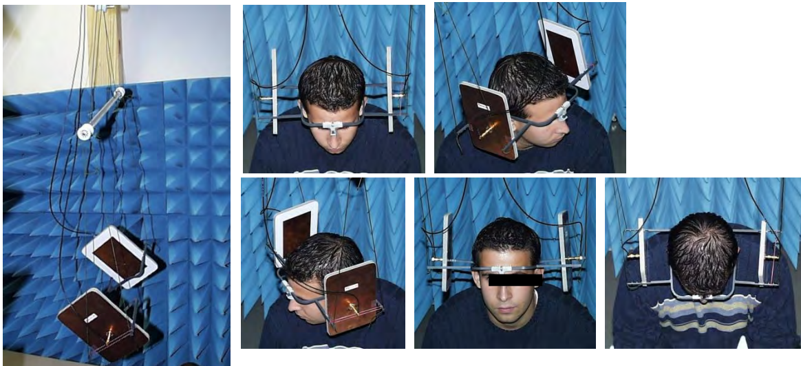
Abbildung 2.9: Durch die Aufhängung des Headsets wird der Proband vom Gewicht der Antennen und der zuführenden HF-Kabel entlastet und es bleibt gleichzeitig eine gewisse Bewegungsfreiheit für den Kopf des Probanden erhalten.
