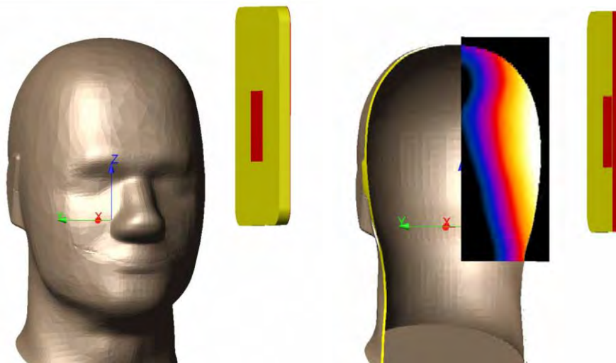
Abbildung 2.33: SEMCAD ® -Modell des SAM-Kopfphantoms bei Befeldung mit der entwickelten 1970 MHz Patch-Antenne (links) und qualitatives Simulationsergebnis (SAR) in der Frontalebene durch den Antennenfußpunkt (rechts)
