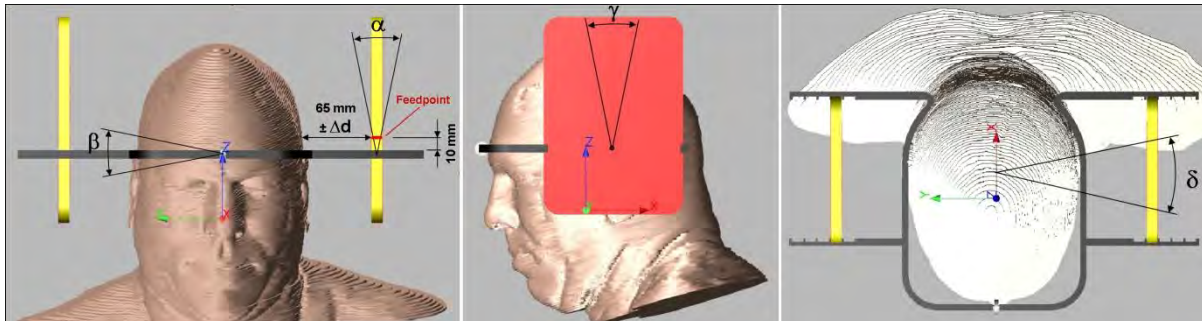
Abbildung 2.12: Definition der Unsicherheitsparameter hinsichtlich der Variation der relativen Lage Antenne/Kopf
